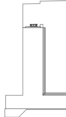
날개벽(우측)
